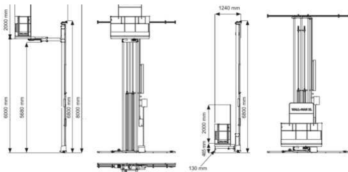
Måttitning - front-, sido- och isovy
