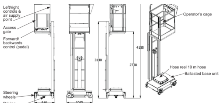
Måttitning – lyfthöjd, bas och räckvidd
